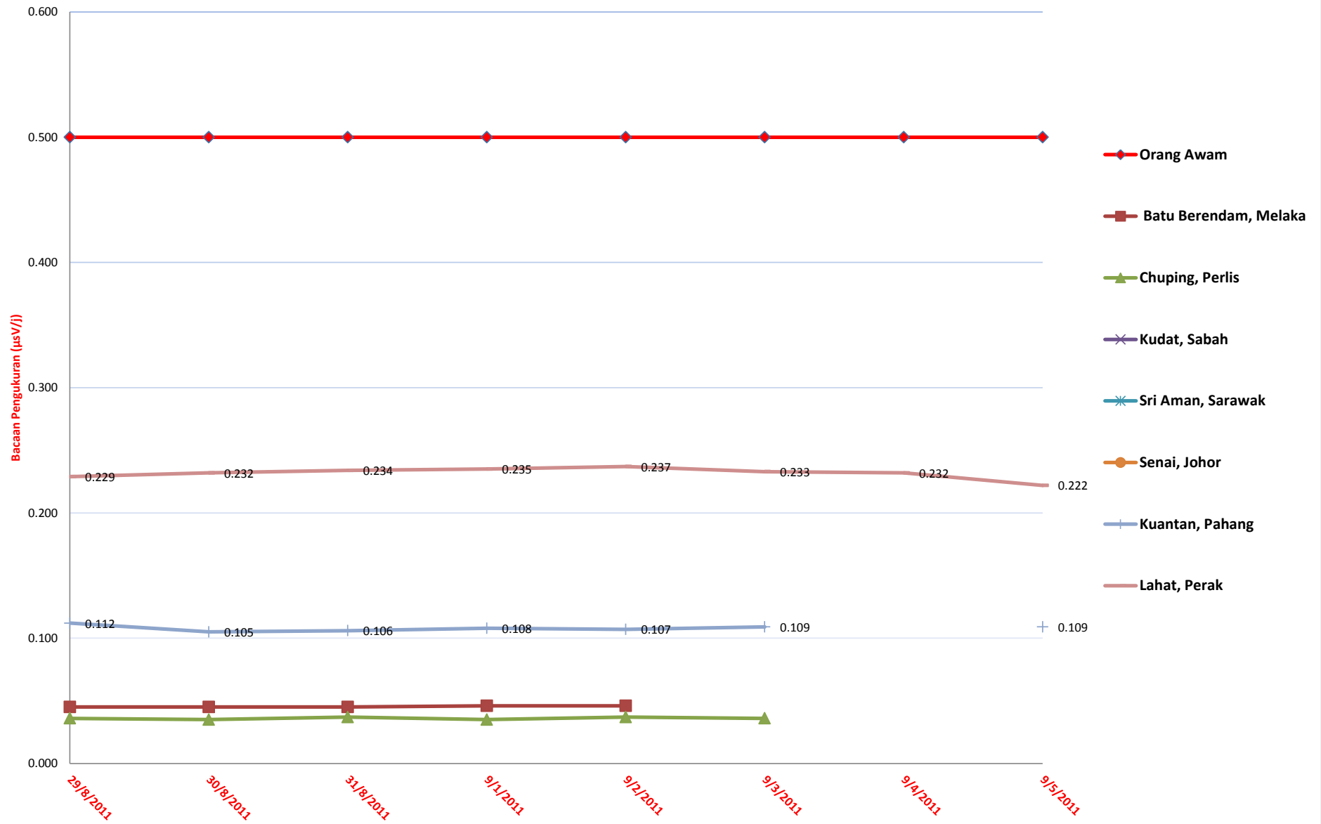
PURATA BACAAN PEMONITORAN ERMS DI TUJUH STESEN MENGIKUT HARI 29 OGOSI 2011 SEHINGGA 5 SETEMBER 2011 ( TOTAL DOSE RATE \mu\text{Sv/h} )
