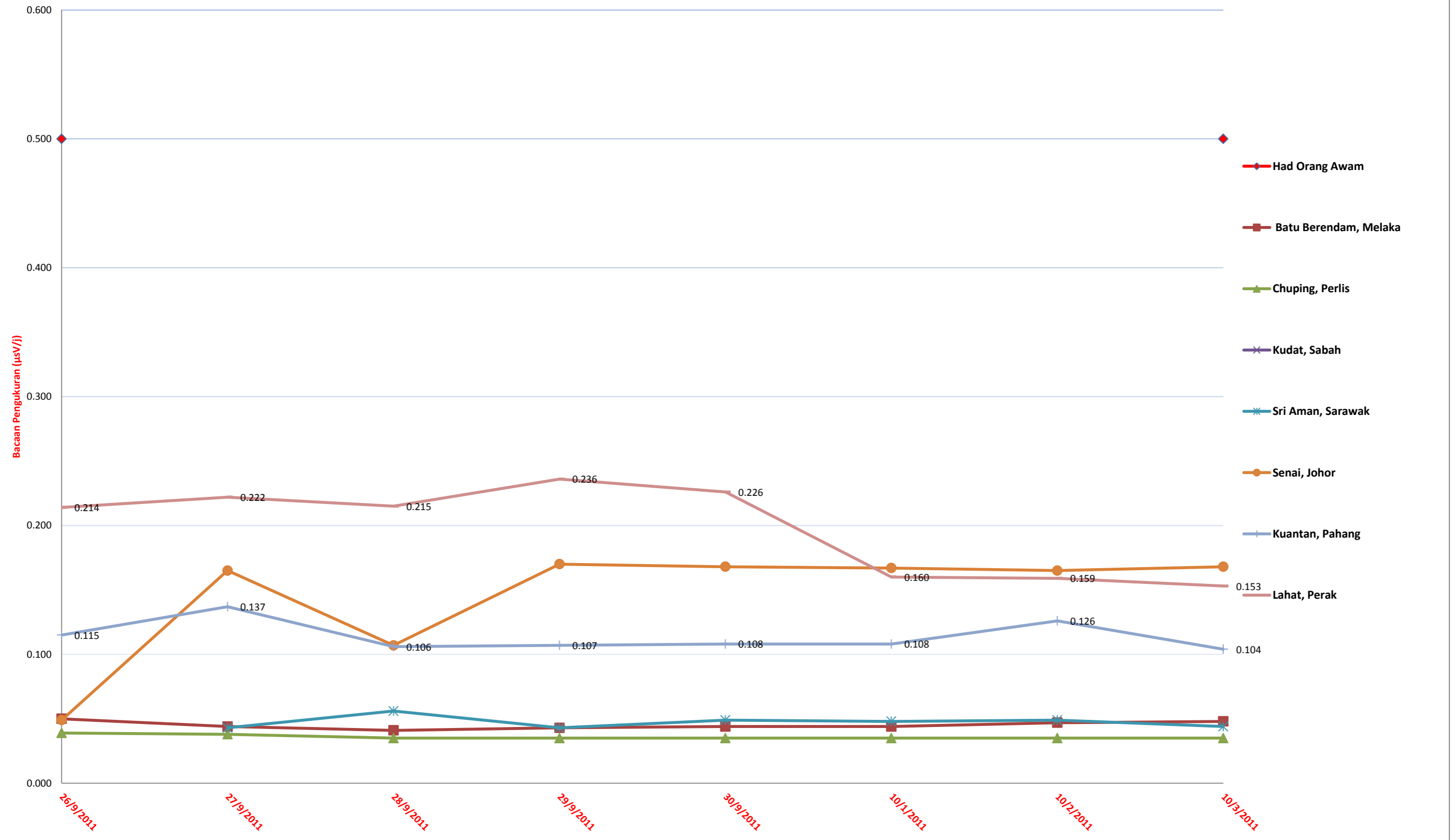
PURATA BACAAN PEMONITORAN ERMS DI TUJUH STESEN MENGIKUT HARI 26 SEPTEMBER 2011 SEHINGGA 3 OKTOBER 2011 ( TOTAL DOSE RATE \mu\text{Sv/h} )
